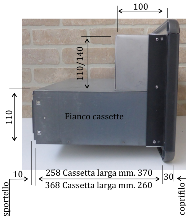
Coprifilo posteriore
